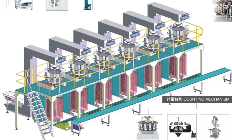
多头秤 Multi-head scale
