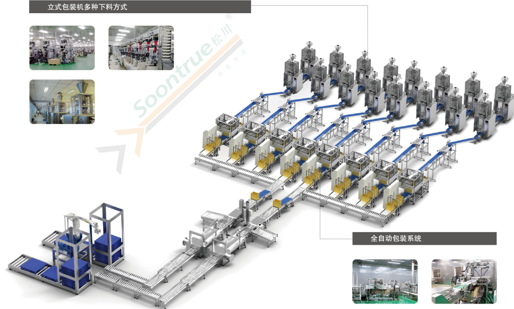
立式包装机多种下料方式
