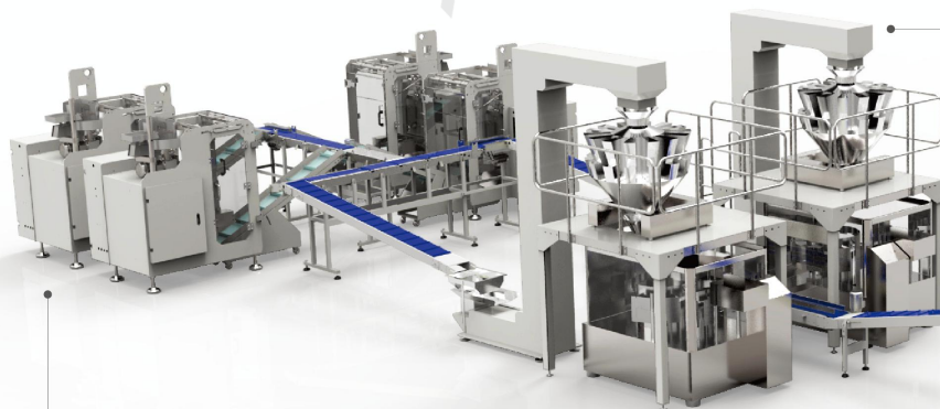
立式小包包装系统
